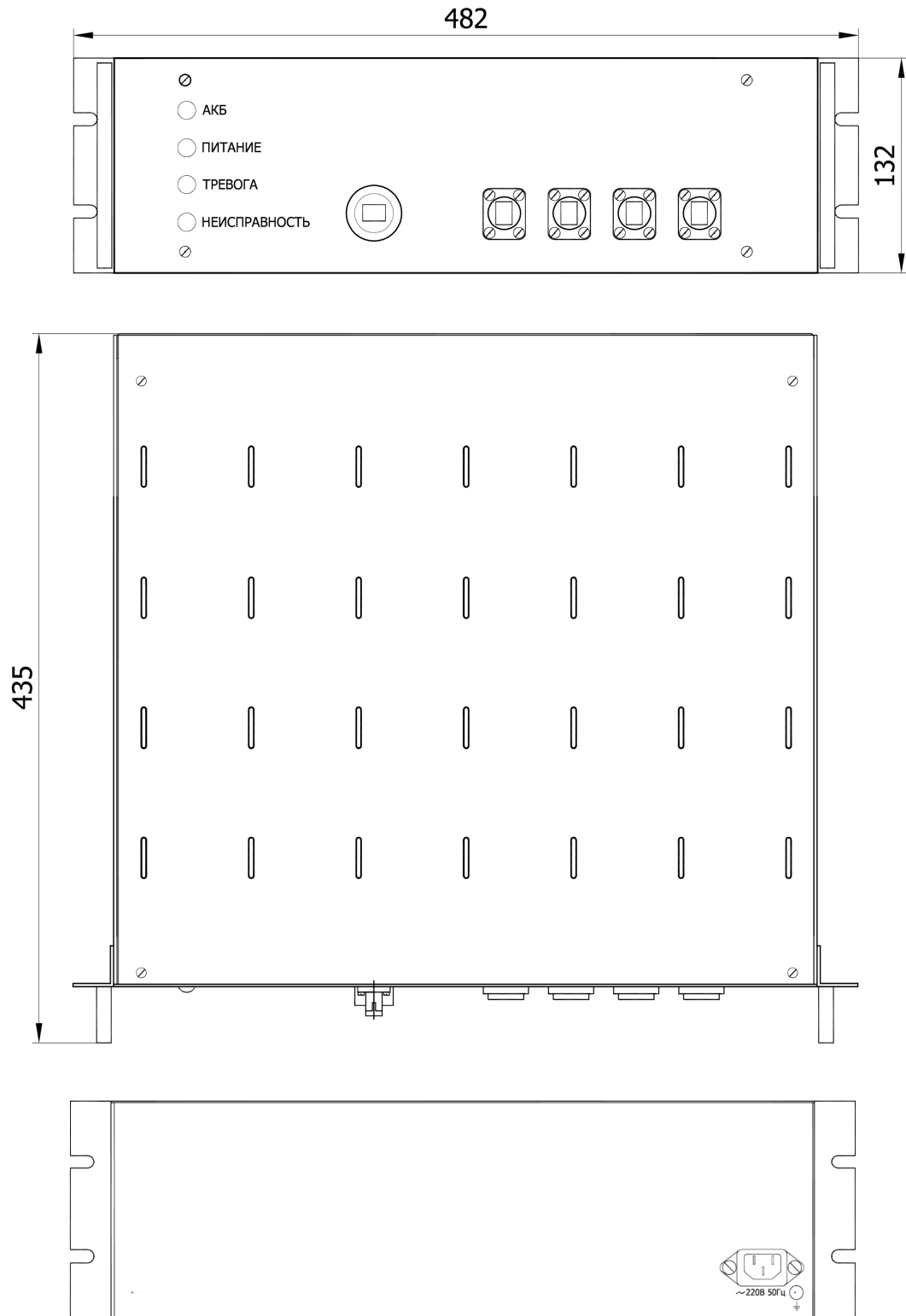
Рисунок 1 - Габаритный чертеж БОС-3-2/19”
